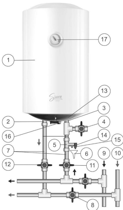
Attēls 1. EŪS pieslēgšana pie ūdensapgādes tīkla
