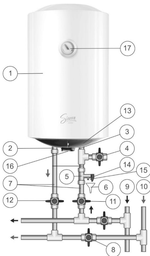
Figure 1: 1 – Chauffe-eau, 2 – Tuyau de connexion de l’eau chaude, 3 – Tuyau de connexion de l’eau froide, 4 – Soupape de purge, 5 – Soupape de sûreté, 6 – Drainage aux égouts, 7 – Tuyauterie d’amenée, 8 – Fermer le robinet d’arrêt pendant l’exploitation du chauffe-eau, 9 – Tuyauterie d’approvisionnement en eau froide, 10 – Tuyauterie d’approvisionnement en eau chaude, 11 – Robinet d’arrêt de l’amenée de l’eau froide, 12 – Robinet d’arrêt de l’amenée de l’eau chaude, 13 – Couvercle de protection, 14 – tuyau d’échappement de la soupape de sécurité, 15 – manche pour ouvrir la soupape de sécurité, 16 – bouton de commande, 17 – indicateur de température.
