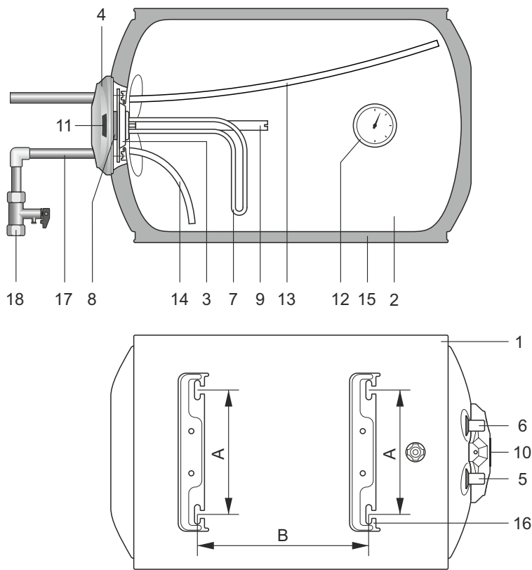
Рис. 2. Горизонтальное размещение
